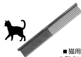
両目櫛 Cat 20×130mm 22g 80針 柄：真鍮 針：炭素鋼 JAN 4969316811983
