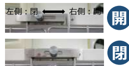
SPマシヨントイプ 扉ラッチ部分 各扉の上下にラッチがあります。 左右の扉を開閉します。
