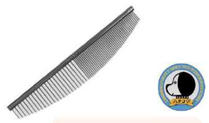
両目櫛 半月型 33×164mm 30g 69針 柄：真鍮 針：ステンレス JAN 4969316815288
