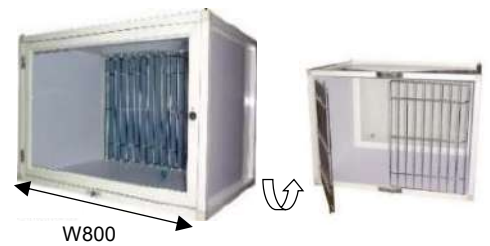
SPS-800 1段 W800×D550×H550 前面扉鍵付強化ガラス(脱着式) 後扉ステンレスネット扉
