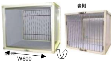
SP-600 1段 W600×D500×H500 前面FIX強化ガラス(はめ込みガラス) 後扉ステンレスネット扉
