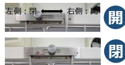
SPマンションタイプ 扉ラッチ部分 各扉の上下にラッチがあります。 左右の扉を開閉します。
